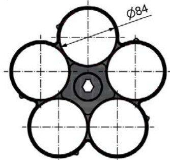
Sez. A-A cups Ø78 - Ø80
