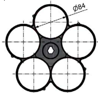
Sez. A-A cups \text{Ø}78 - \text{Ø}80
