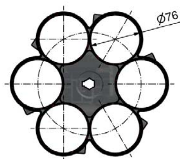
Sez. A-A
